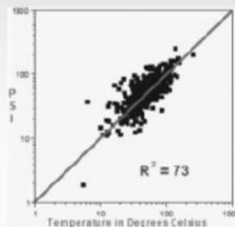
散点图
