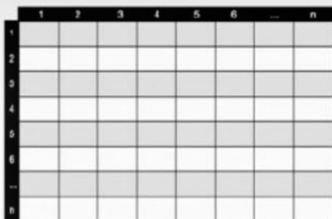
矩阵图
