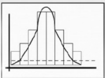
直方图
