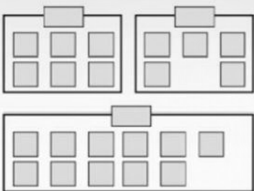
亲和图
