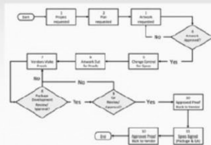
流程图
