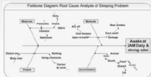
因果图
